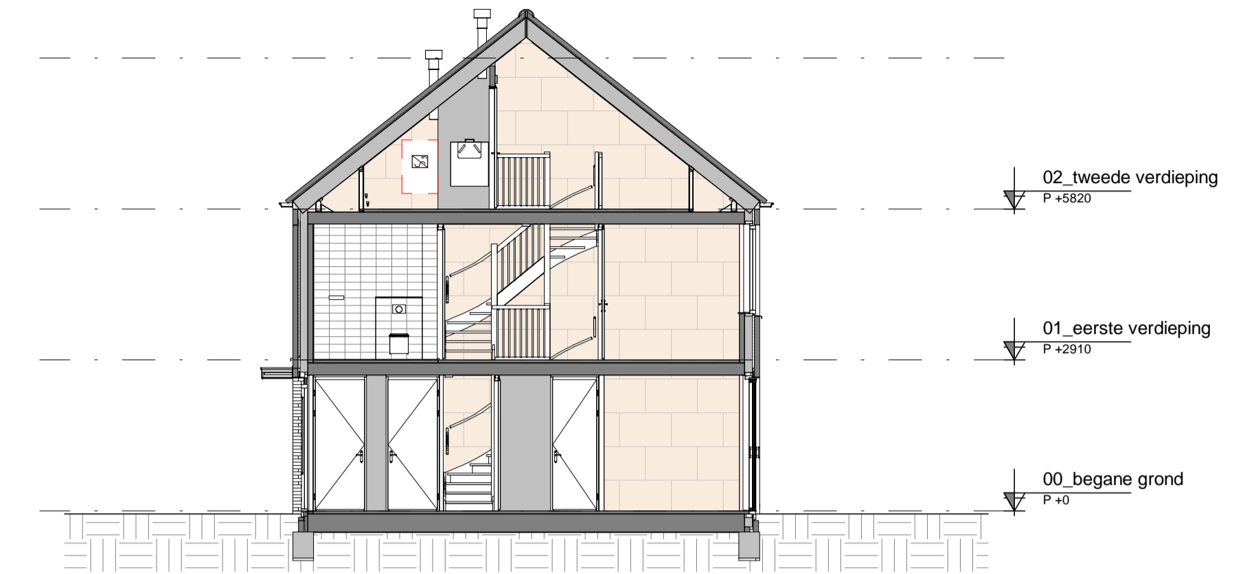
Doorsnede D.A
