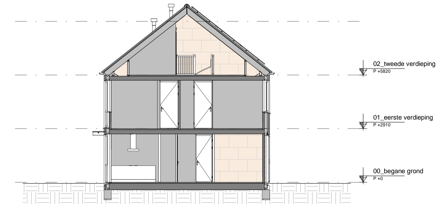
Doorsnede D.B
