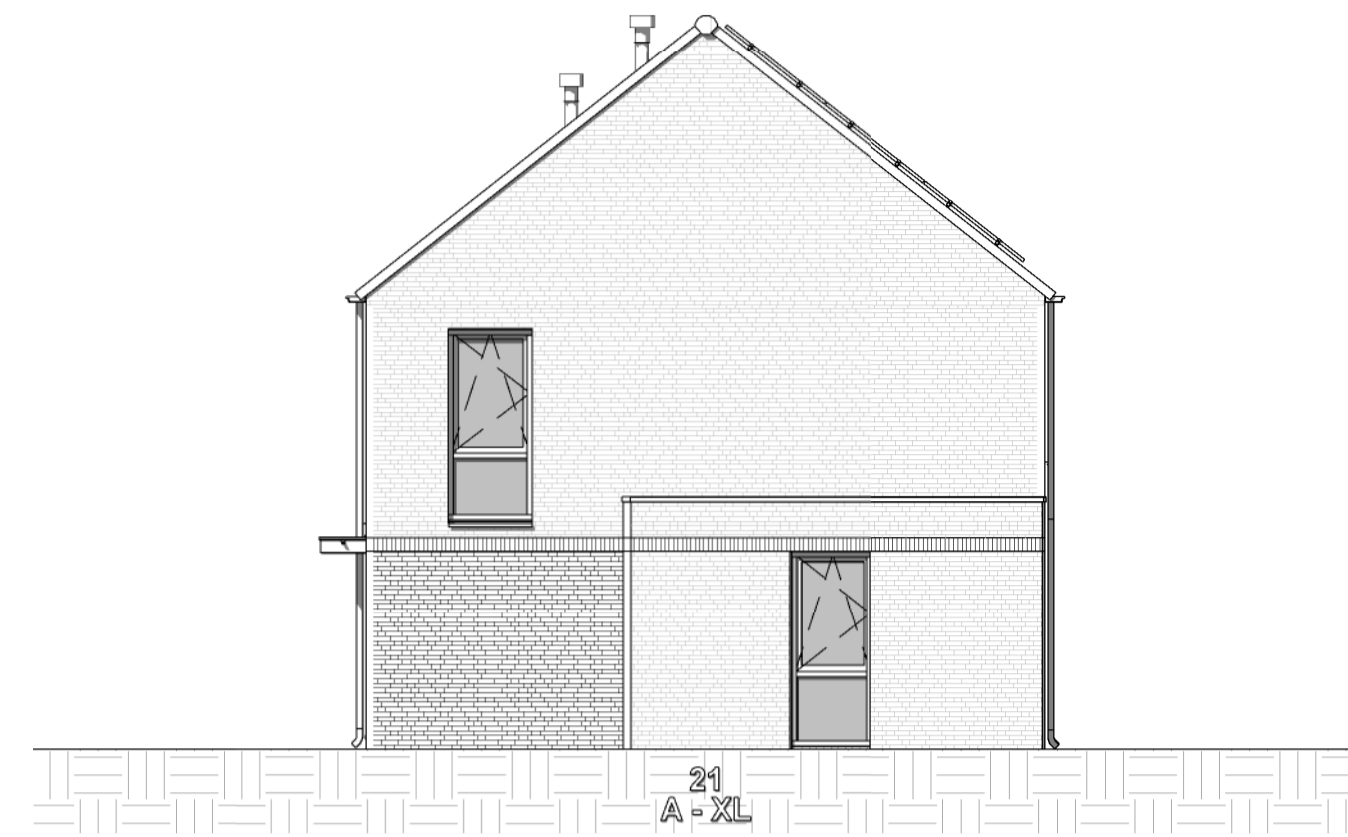
Rechterzijgevel
