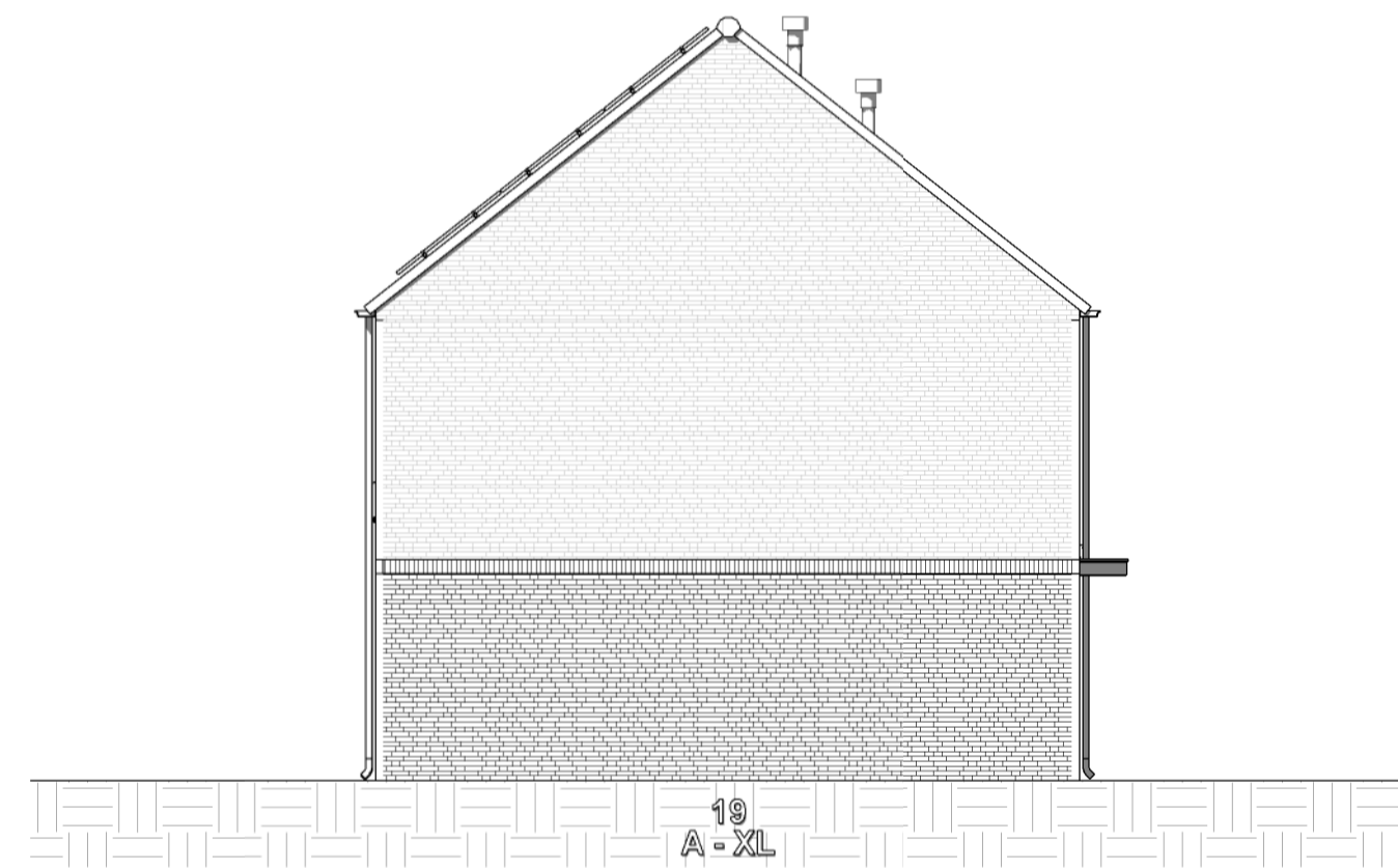
Linkerzijgevel
