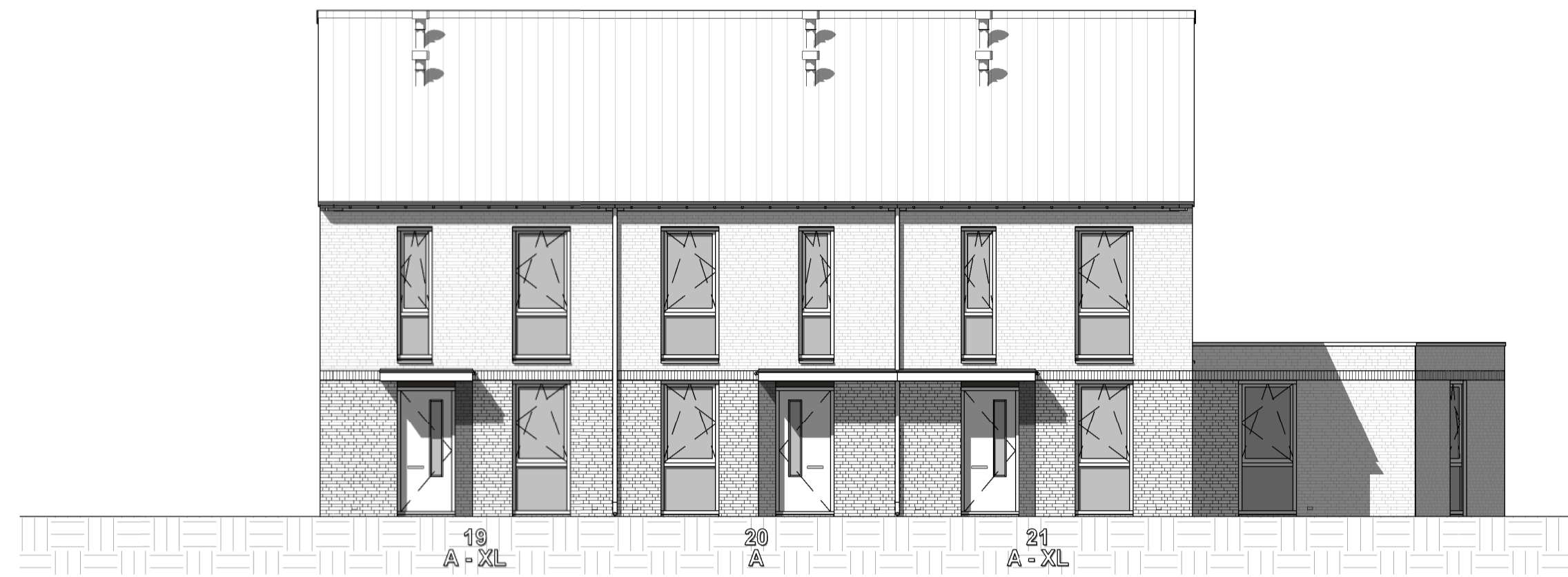
Voorgevel
